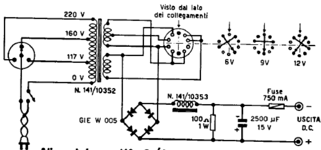
Alimentatore N° 2/1
